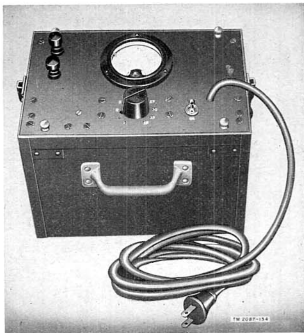
Figure 32. Decibel Meter TS-399/U.
